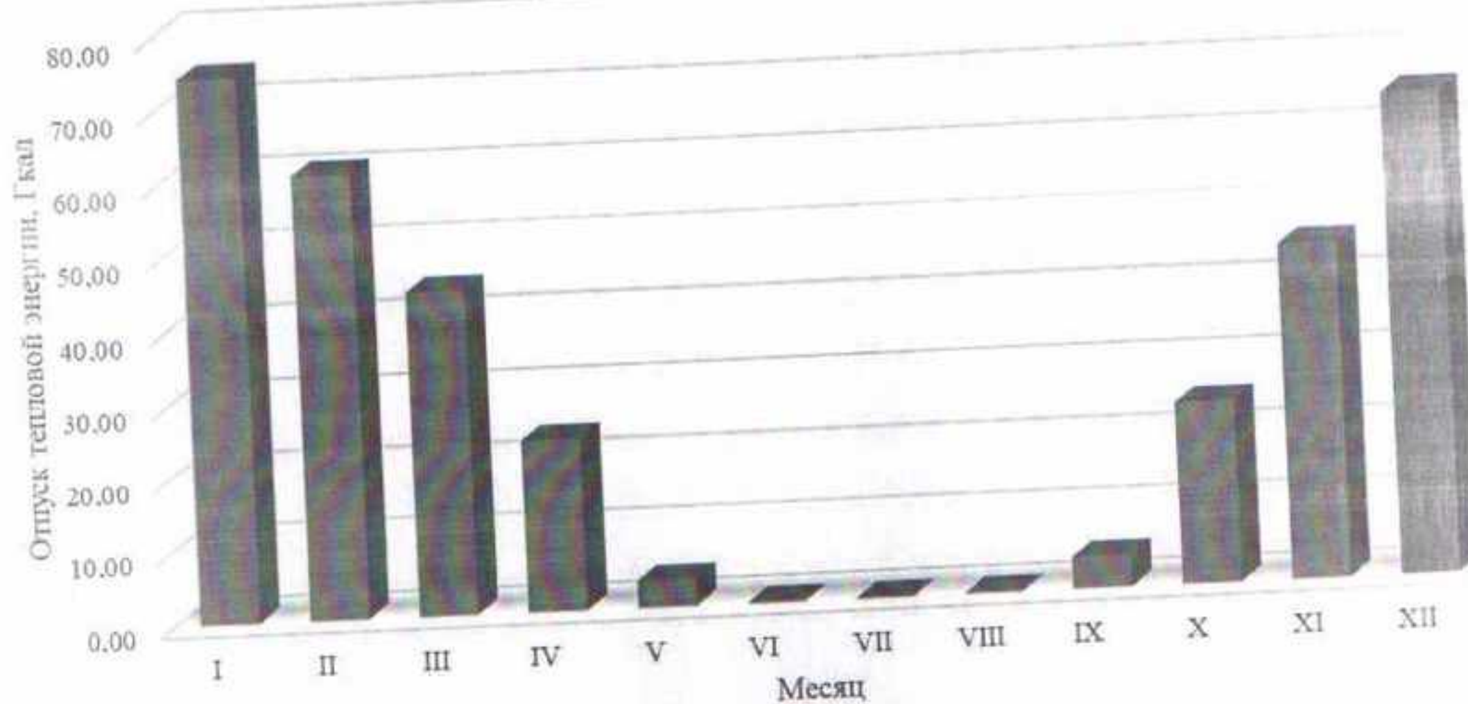
Рисунок 1.2 – Оптимальный температурный график отпуски тепловой энергии по котельной с. Новоникольское
